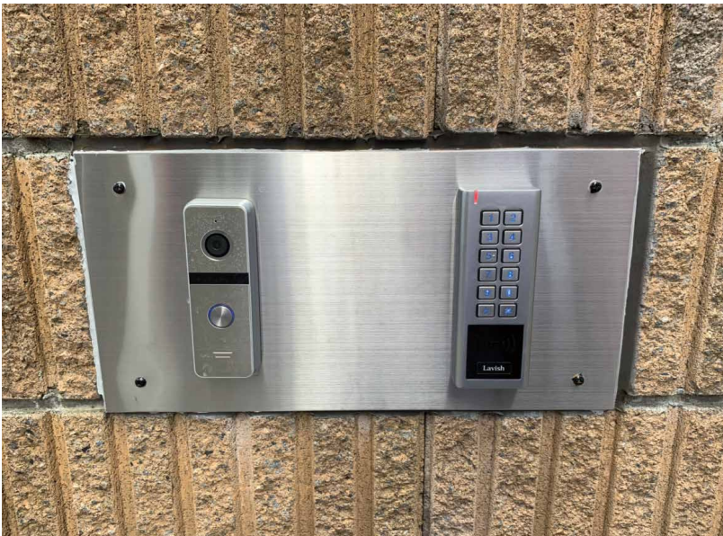
メインゲートインターホン (V-K1 / RER-SKX5EHM / 居室にはV-M1を設置)
