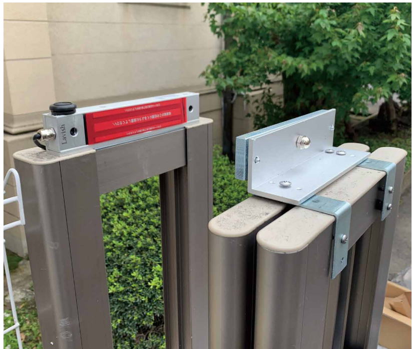
アコーディオン門扉へ設置 (LOEW-B280L / BR-B280-ZL)
