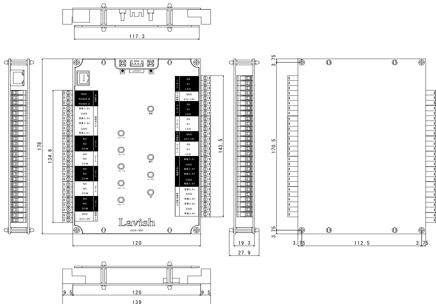
【COA-45F 寸法図】
