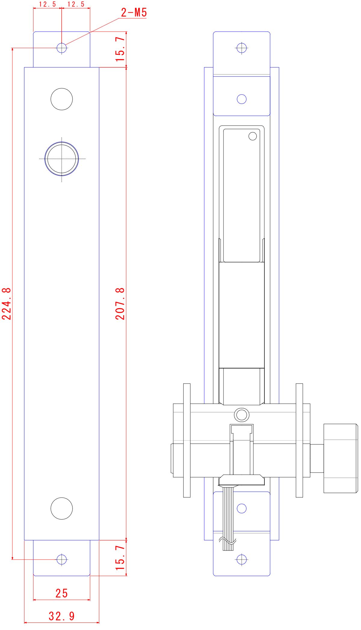
【本体・フロントプレート・カバープレート・シリンダー組み立て後】
