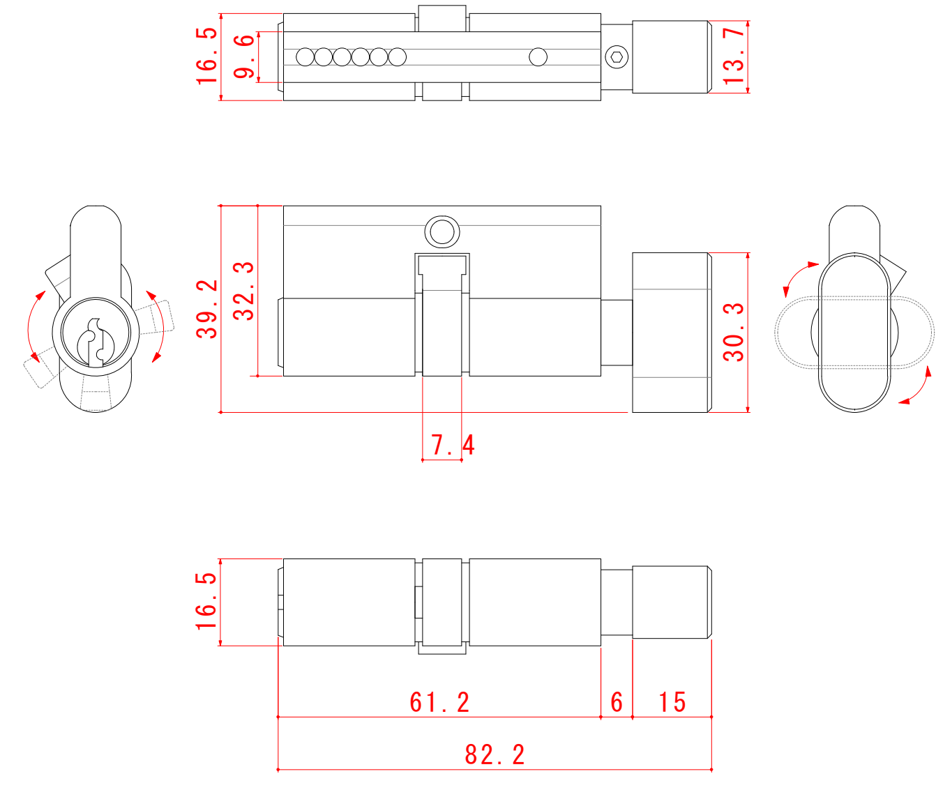
【シリンダー】
