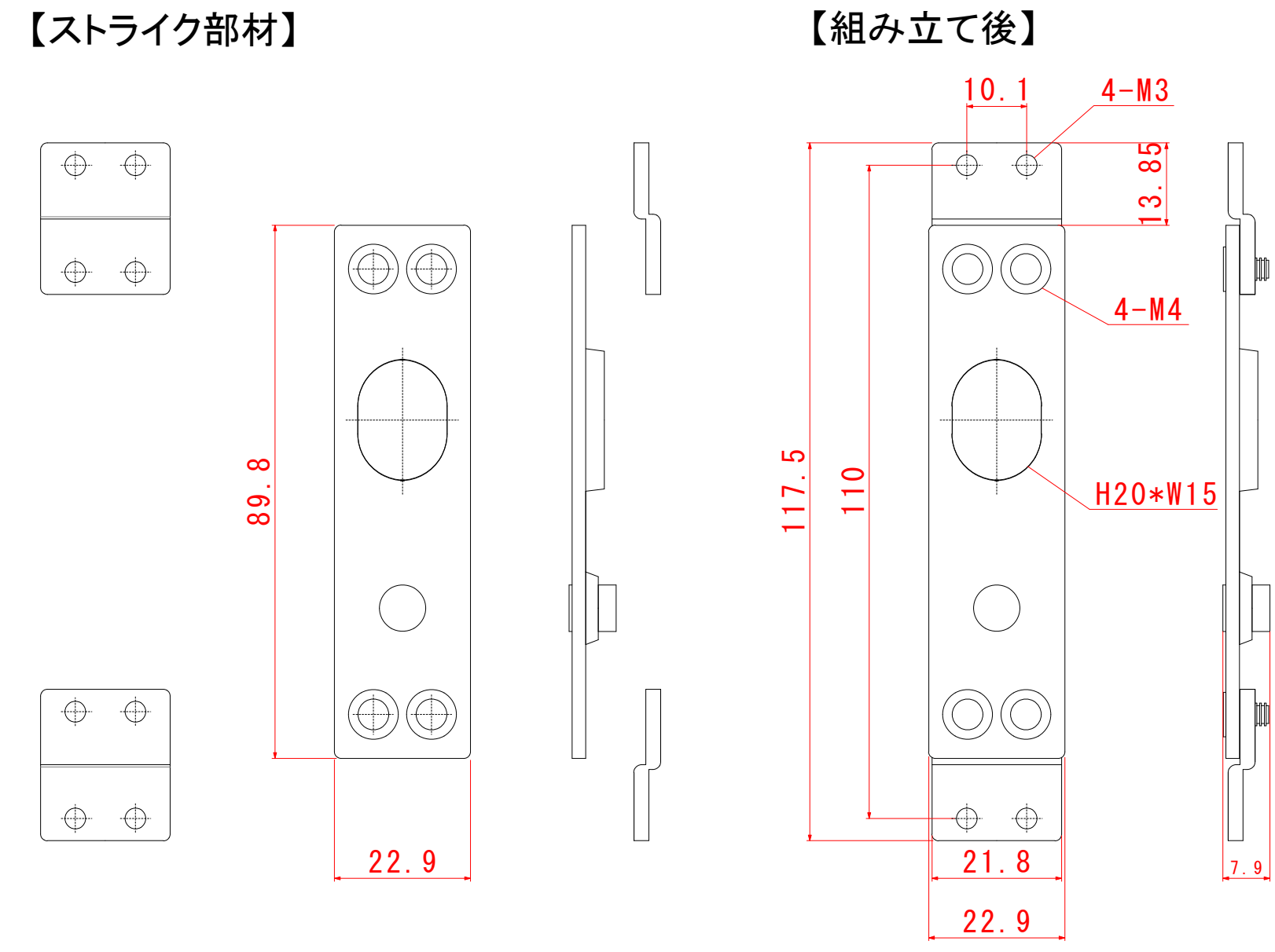
【ストライク】
