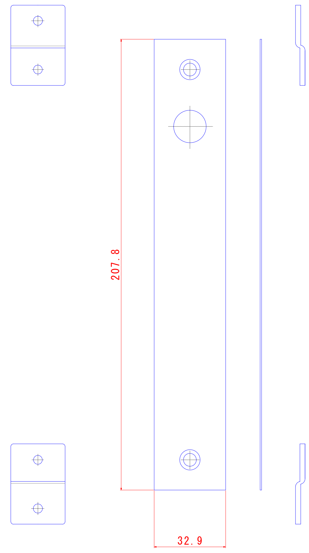
【フロントプレート】
