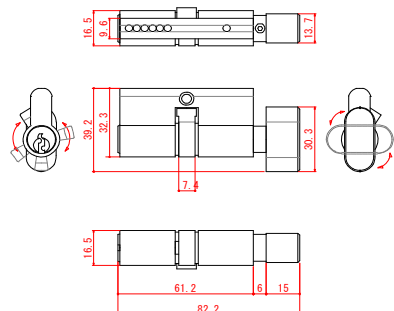
【シリンダー】
