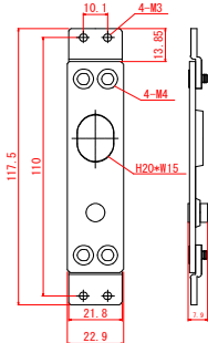
【組み立て後】
